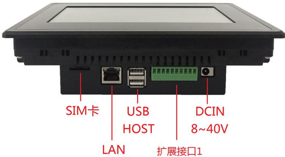
下侧接口
