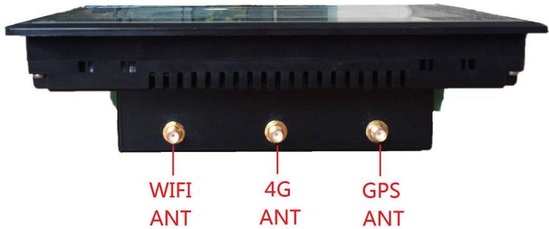
上侧接口
